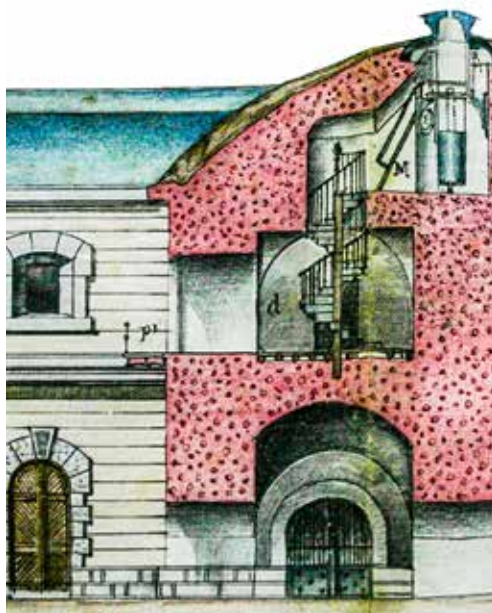
d: estancia anexa al observatorio (existente). M Observatorio acorazado (inexistente) al que se accede desde el centro de la estancia d por medio de una segunda escalera de caracol. Se observa el vano hacia el patio de infantería.
