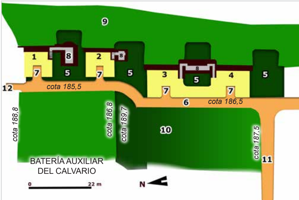
1, 2, 3, 4 Asentamientos de artillería. 5 Traveses. 6 Terraplén de servicio, ligeramente rehundido. 7 Rampas. 8 Repuestos de munición. 9 Parapeto. 10 Terreno en ligera pendiente. 11 Camino de acceso a la batería. 12 Acceso al camino cubierto del fuerte de Guadalupe. La zona próxima (10) a la batería parece diseñada para proteger la gola de la batería.
