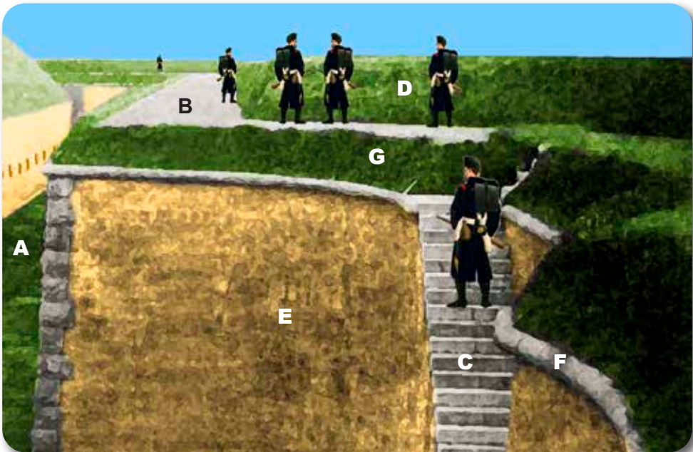
Reconstrucción del entorno original del camino cubierto: A Foso. B camino cubierto en su disposición original, en el tramo correspondiente a la caponera de gola. En primer plano ( C ) una de las escaleras de contraescarpa. Se observa el piso totalmente plano de arena mezclada con gravilla; El parapeto ( D ), dotado de un ligero talud, está cubierto de hierba. E contraescarpa, F cordón, G talud entre el cordón y el camino cubierto.
