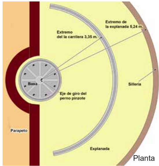
Explanada genérica para un cañón de hierro entubado de 15 cm «Ordóñez», en marco alto. Imagen superior: planta. Imagen inferior: sección.
