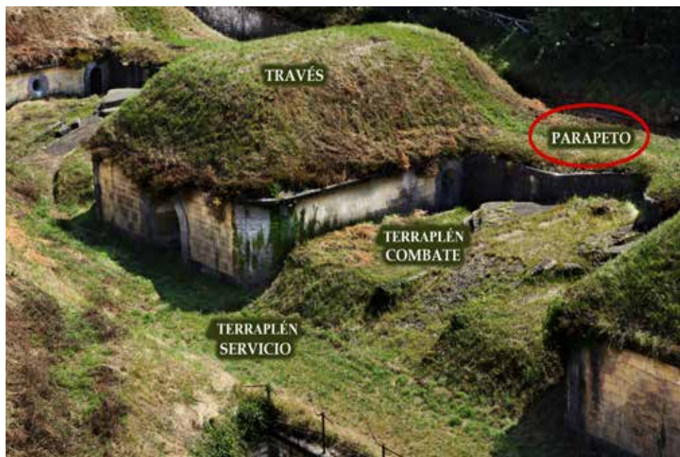
Sector de parapeto de la Obra del Centro. La rotulación indica su relación con los terraplenes) de combate y de servicio.
