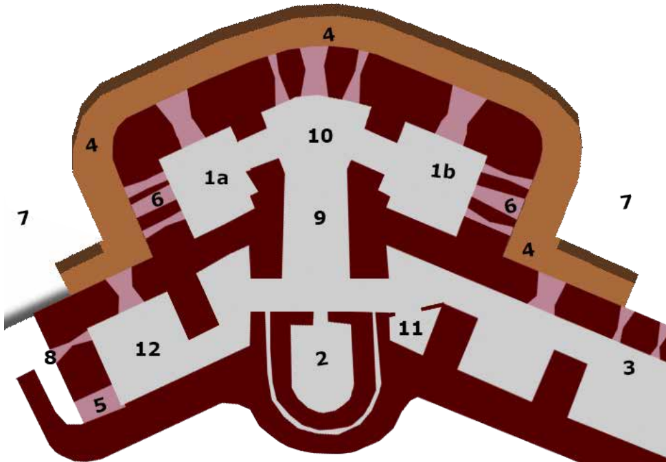
Plano de la caponera suroeste: 1 Casamata de flanco. 2 Repuesto. 3 Galería de escarpa. 4 Refosete. 5 Puerta del camino de ronda. 6 Cañonera de flanco. 7 Foso 8 Aspillera del camino de ronda. 9 Bóveda de comunicación de las dos casamatas. 10 distribuidor a las casamatas. 11 Letrina
