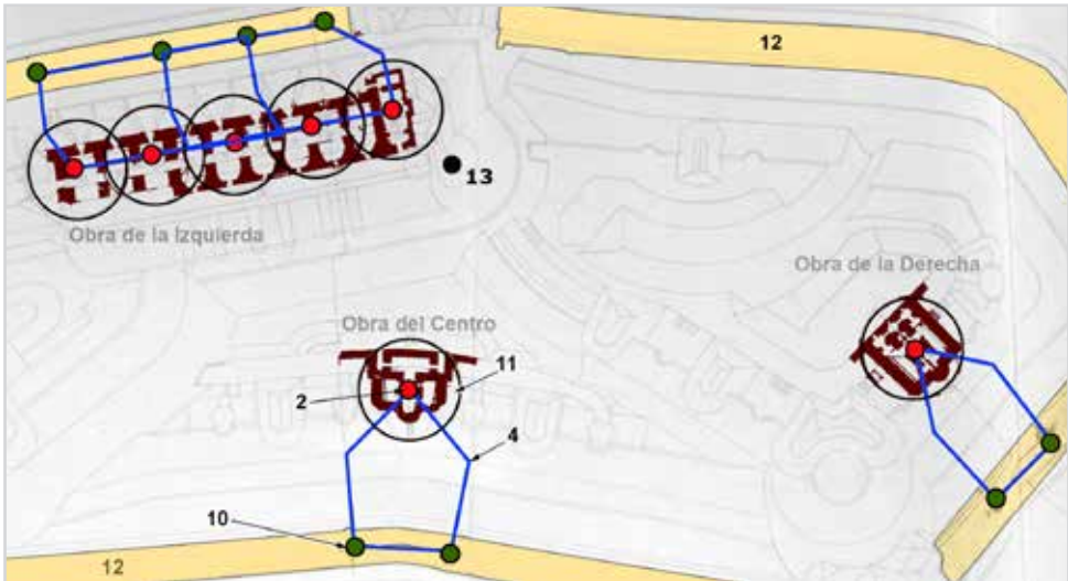
Esquema del sistema de pararrayos según el Proyecto (1906): 2 Barra. 4 cables conductores. 10 Dispersadores. 11 Zona teóricamente protegida por el pararrayos. 12 Foso. 13 situación inicial del asta de bandera y del primer y único pararrayos hasta 1906.
