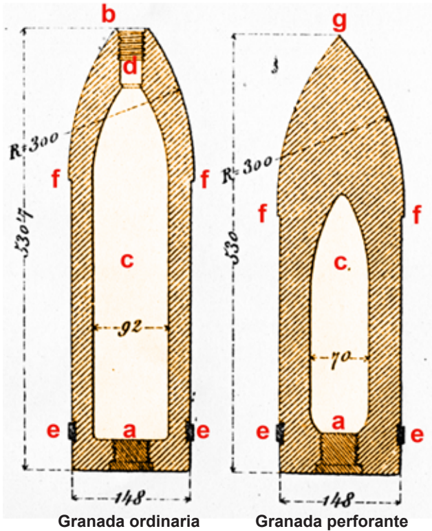
PROYECTILES PARA EL CHE 15 CM «ORDÓÑEZ» mod. 1885
