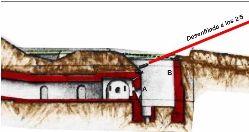
En el Proyecto se aprecia que la caponera (A) es más baja que la contraescarpa (B).
