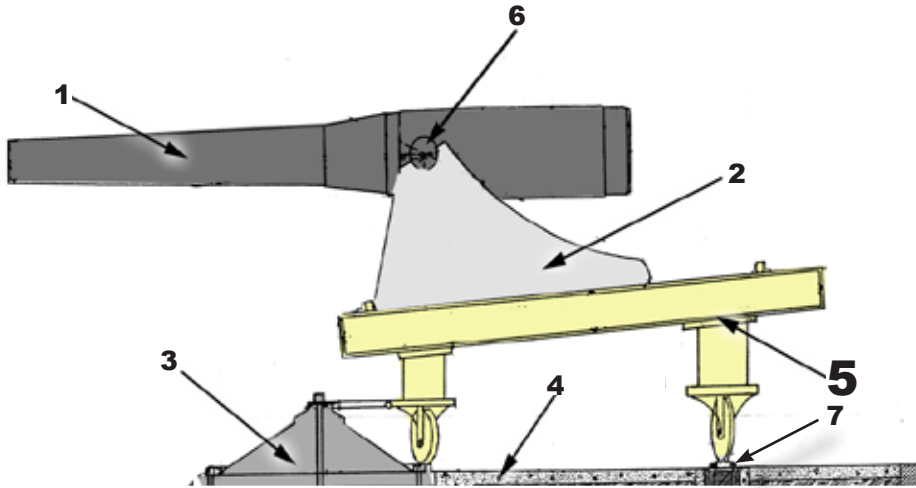
Esquema de la disposición del tubo, cureña y marco en un Cañón de Hierro Entubado «Ordóñez» de 15 cm, mod. 1885, sobre «marco alto». 1 Tubo. 2 Cureña. 3 Basacarril. 4 Explanada. 5 MARCO. 6 Muñones. 7 Carrilera trasera o carrilera de contera.
