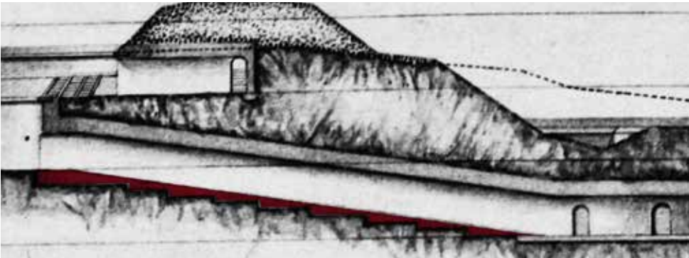
Cimientos (en rojo) de la poterna de la caponera de la Obra de la Derecha
