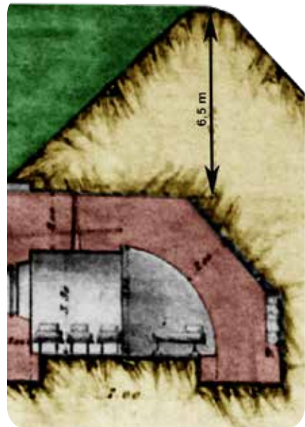
Blindaje de (6,5 m) sobre el trasdós de las bóvedas del cuartel de artillería, según el proyecto del fuerte (coloreado no original).
