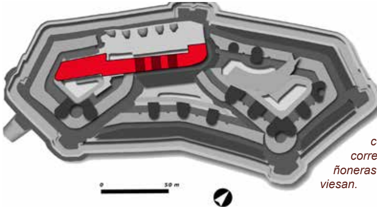
Obra de la Izquierda. La máscara o espaldón se ha coloreado en de rojo. El sector oriental (derecha de la fotografía) se utiliza actualmente como mirador en las visitas turísticas del Fuerte, cuyo acceso fue posible mediante la formación de una nueva rampa de acceso.
