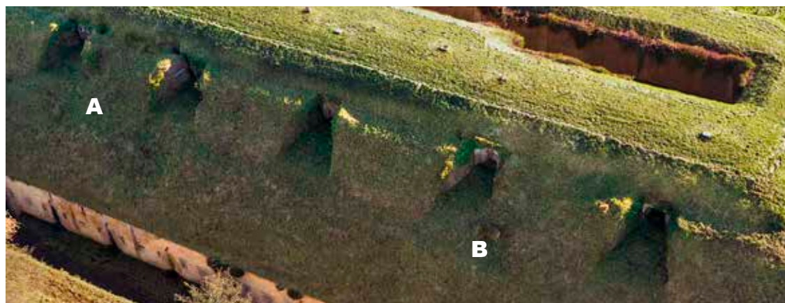
Frente norte de la batería acasamatada con las cinco cañoneras abiertas y los dos desprendimientos (A y B) del blindaje actualmente existentes, acompañados de daños en el hormigón de de las derivas de las cañoneras Pudieron ser causados bien por los rebufo de los disparos propios o bien por impactos de proyectiles enemigos en los combates de 1936.
