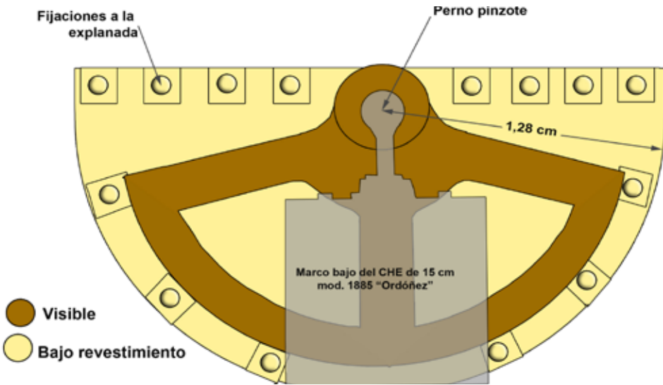
Estructura de una basacaril para marco bajo de un CHE de 15 cm «Ordóñez» mod. 1885.
