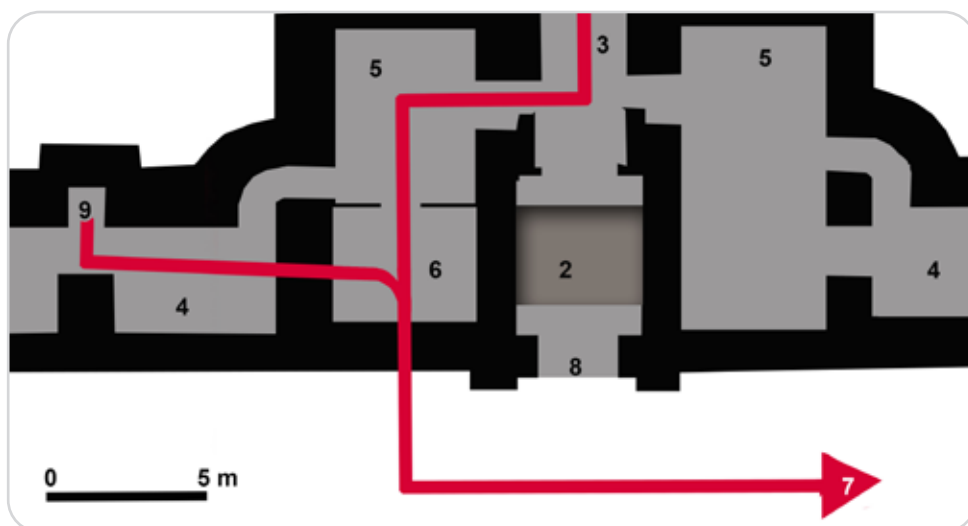
Esquema de la red de saneamiento a su paso por la puerta principal. 1 Foso. 2: Foso de la puerta principal. 3: Poterna de acceso al patio principal. 4: Galería de escarpa. 5: Cuerpo de guardia de la puerta principal. 6: Casamata para batir la puerta de acceso al foso. 7: Red de saneamiento. 8 Puerta principal. 9 WC. Nótese el desvío que realiza la red de saneamiento para salvar el foso de la puerta principal (2), que sirve como ejemplo para ilustrar su nula coincidencia con lo previsto en el Proyecto.
