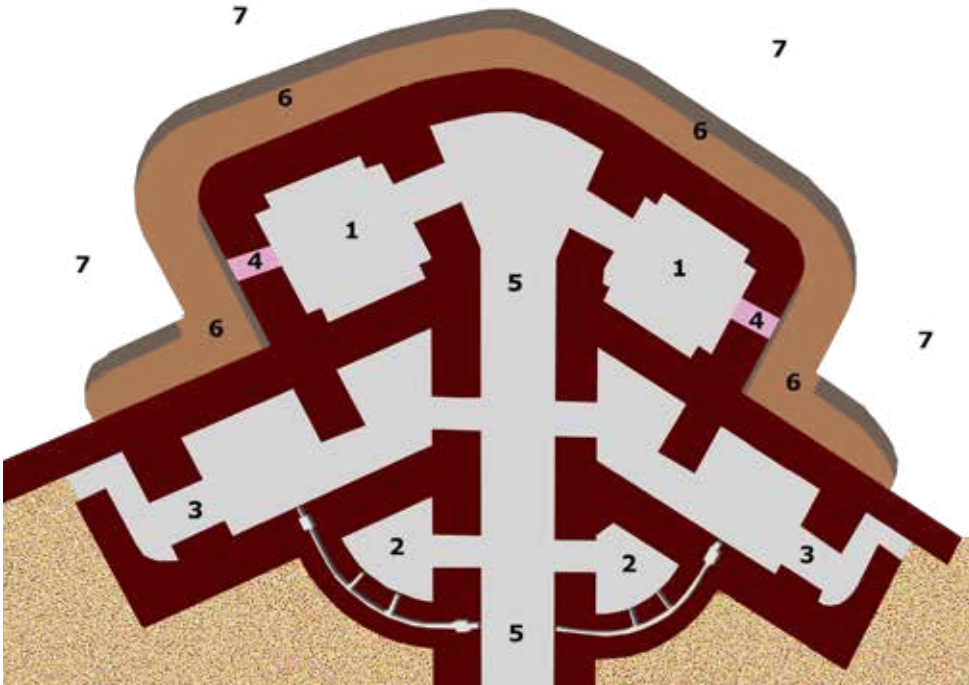
Plano de la caponera sureste: 1 Casamata de flanco. 2 Repuesto. 3 Puerta del camino de ronda. 4 Cañonera de flanco. 5 Poterna de acceso desde el patio Oriental. 6 Refosete 7 Foso. (No se han incluido 8 aspilleras, 5 matacanes con sus banquetas y 8 lanzagranadas).
