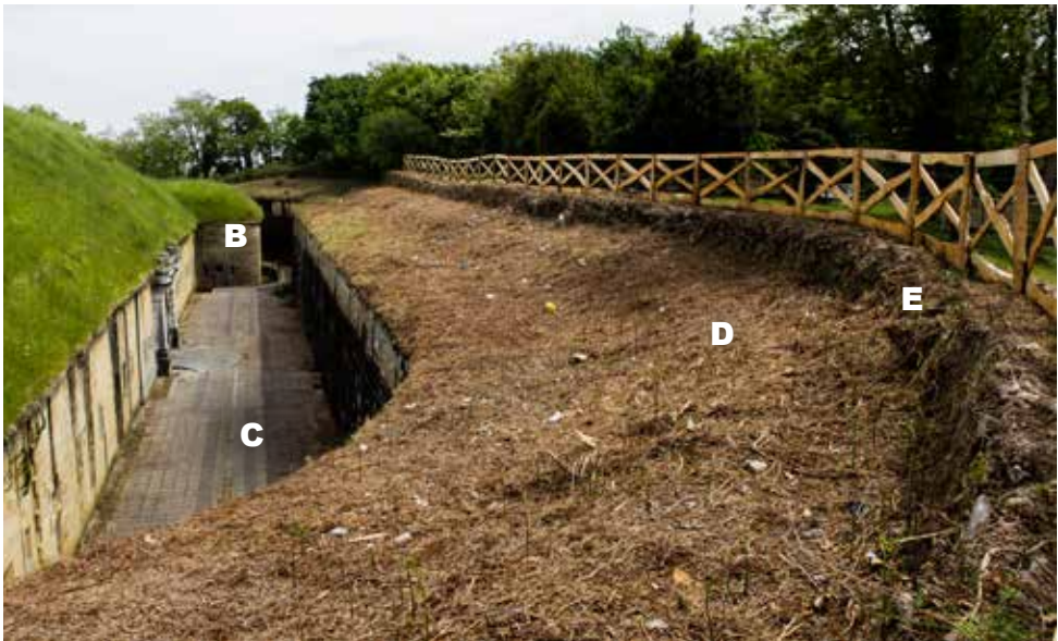
Camino cubierto en el entorno de la caponera suroeste ( B ). Se aprecia el foso ( C ), así como una banqueta ( D ) de tierra que, entre la citada caponera y la semicaponera SW, facilitaba el disparo de los soldados desde el parapeto ( E ), en este sector revetido de mampostería.
