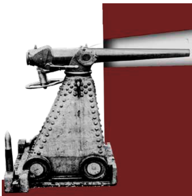
Disposición de un cañón Nordenfält con montaje de caponera en una cañonera. La explanada es pequeña y sirve para retener las ruedas e impedir el movimiento de retroceso del cañón en el momento del disparo. En el ángulo inferior izquierdo se observa un cartucho.
