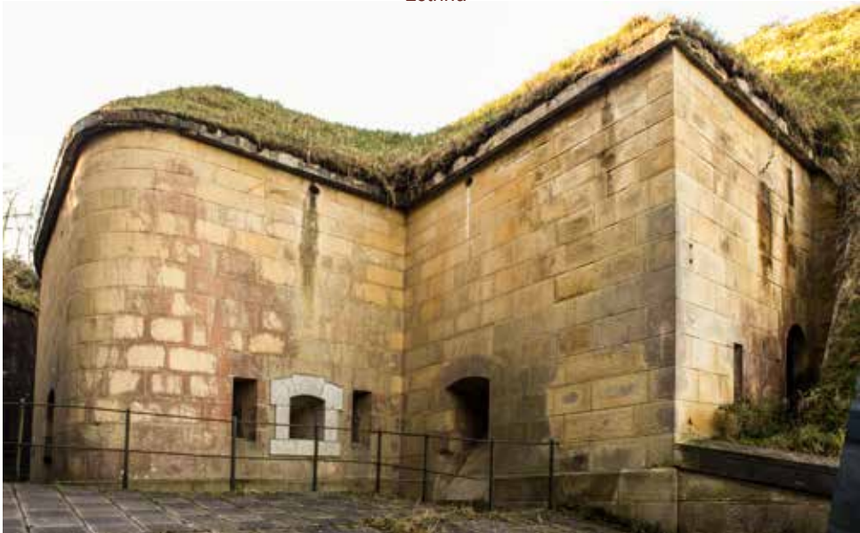
Frente oriental de la caponera suroeste. Se observa la cañonera y las dos aspilleras del frente, así como un matacán para defensa del fosete. A la derecha, la puerta de acceso al camino de ronda de la escarpa.
