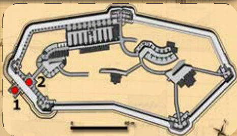
Puentes móviles sobre fosos de acceso: 1 Puente de la antepuerta. 2 Puente de la puerta principal.
