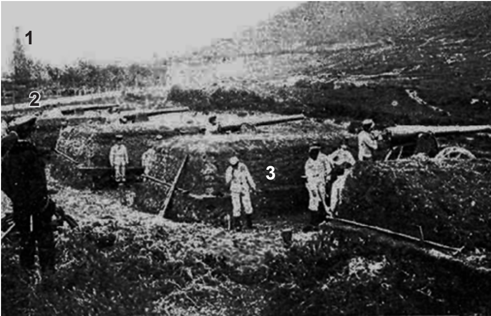
1: Chapitel del Santuario de Guadalupe. 2: Camino militar al Fuerte. 3 Través de la batería de prácticas. Las piezas que artillan la batería en ese momento (noviembre de 1905) son 4 cañones de bronce de 12 cm «Plasencia» con objeto de disparar hacia el mar, ya que era más complicado hacer prácticas disparando hacia tierra (Nuevo Mundo ).
