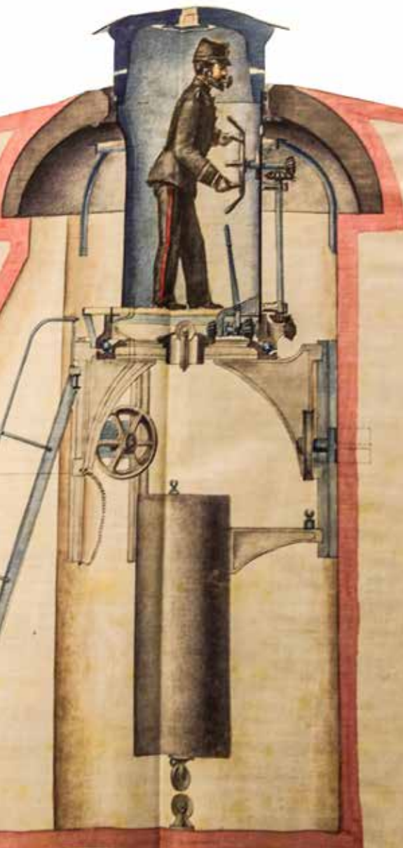
Proyecto no ejecutado de un observatorio acorazado eclipsable para el fuerte de Guadalupe (1899).
