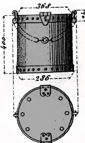
Cubo para lubricante
