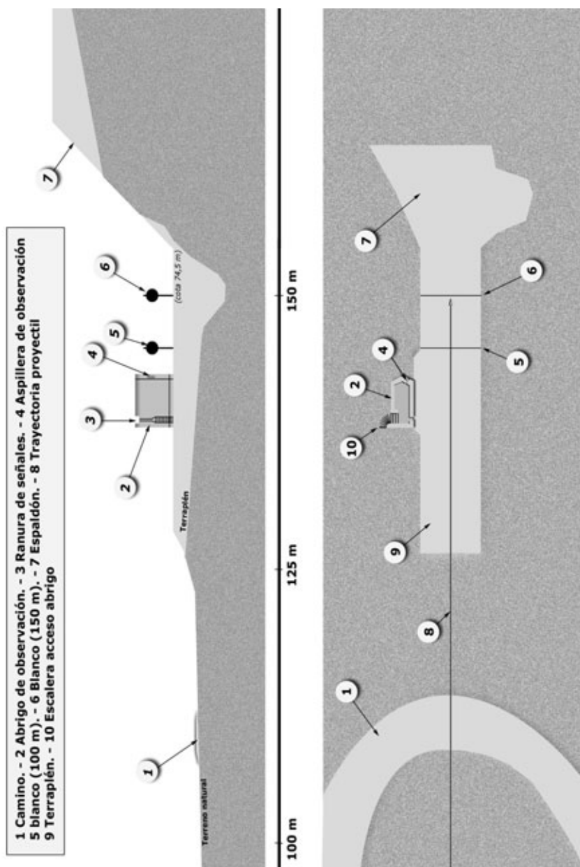
Galería de tiro. Estado en 1916. Sector occidental
